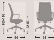
DU103/DU203 Poltrona direzionale con braccioli e oscillante mov.27 tilting. Directional armchair with mov.27 tilting.
