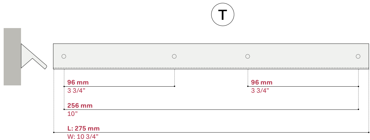
Maniglia per ante piene, vetro acidato o vetro retrolaccato con telaio in alluminio / Handle for wooden doors, acetated or rear-lacquered glass with aluminium frame
