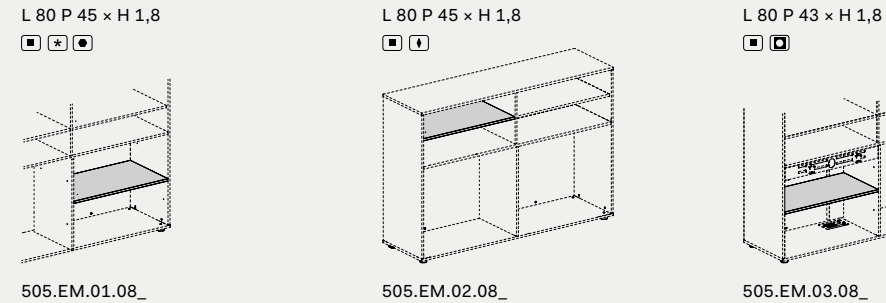
505.EM.01.08_ L 80 P 45 x H 1,8 505.EM.02.08_ L 80 P 45 x H 1,8 505.EM.03.08_ L 80 P 43 x H 1,8
