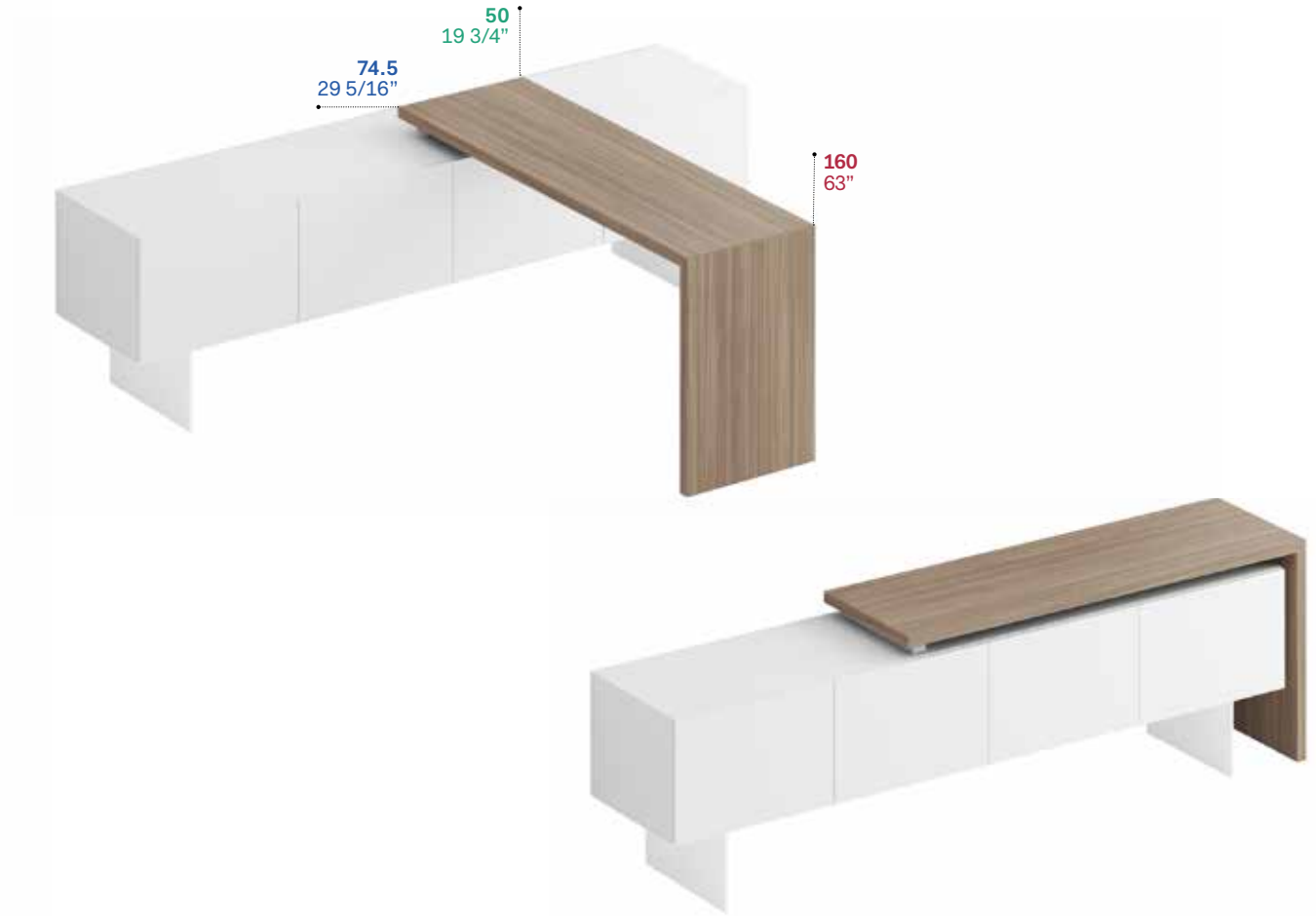
Posizione 1 / Position
