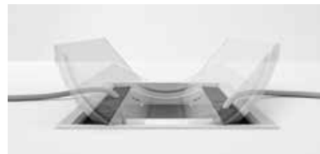
Top access con integrazione multipresa elettrica / Top access with electrical socket integration
