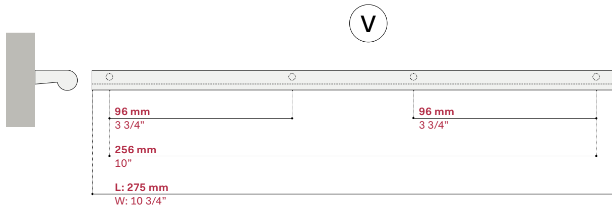
Maniglia per ante piene, vetro acidato o vetro retrolaccato con telaio in alluminio / Handle for wooden doors, acetated or rear-lacquered glass with aluminium frame
